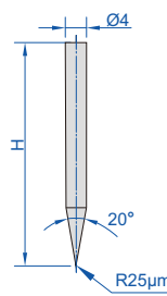
cone stylus
