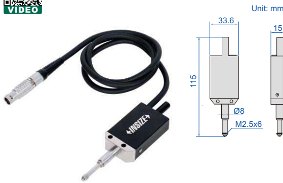
linear gage 7131-01
